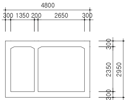
< 단면 11-11 >
