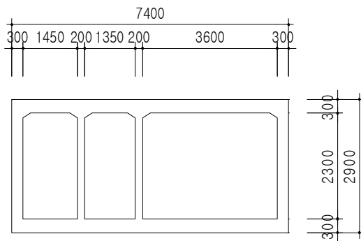
< 단면 9-9 >
